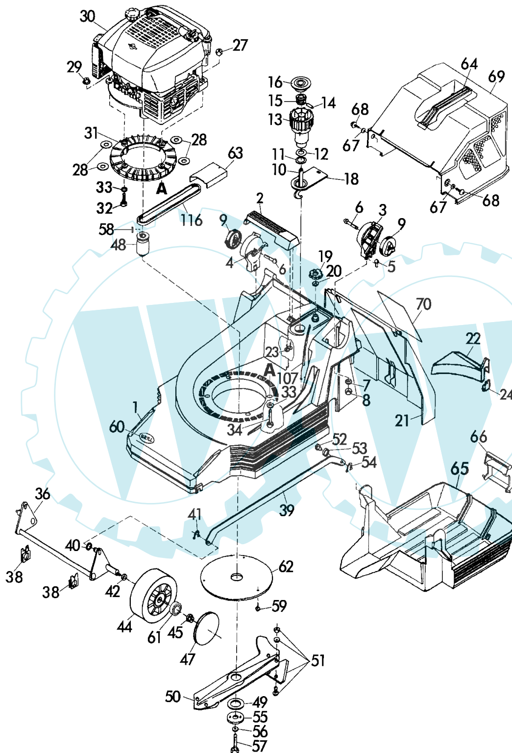
40 BR V12 - Art.78575 ab Baujahr 1995
